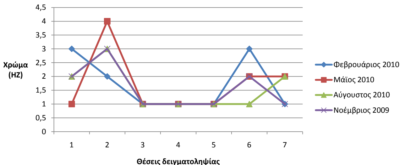
Διάγραμμα 9-Παραρτήματα 1.1-1.2.α-1.2.β-1.2.γ Τιμές χρώματος δειγματοληψίας Μαΐου 2010 και δειγματοληψιών Νοεμβρίου 2009, Φεβρουαρίου, Αυγούστου 2010 που πραγματοποιήσε το εργαστήριο περιβαλλοντικής επιστήμης και τεχνολογίας
