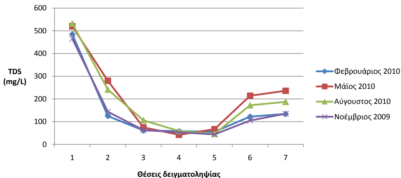
Διάγραμμα 21-Παραρτήματα 1.1 - 1.2.α - 1.2.β - 1.2.γ Συγκεντρώσεις ολικών διαλυμένων στερεών δειγματοληψίας Μαΐου 2010 και δειγματοληψιών Νοεμβρίου 2009, Φεβρουαρίου, Αυγούστου 2010 που πραγματοποίησε το εργαστήριο περιβαλλοντικής επιστήμης και τεχνολογίας
