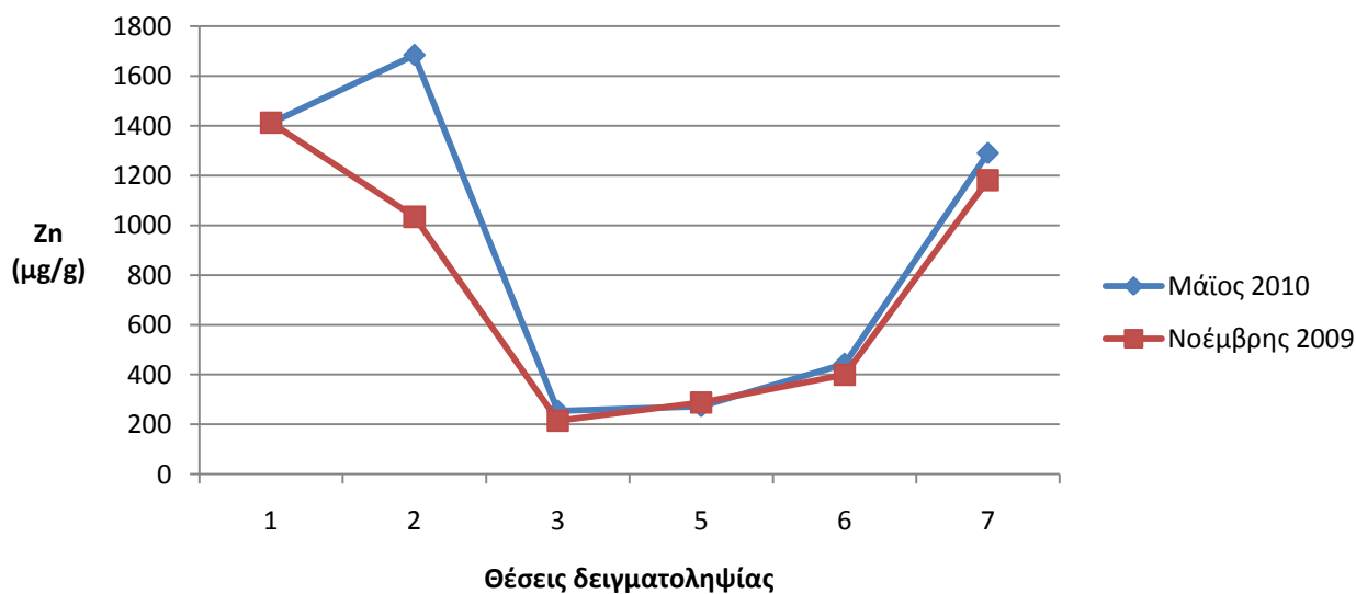
Διάγραμμα 63-Παράρτηματα 2.1 - 2.2 Συγκεντρώσεις ψευδάργυρου από δειγματοληψία Μαΐου 2010 και από δειγματοληψία Νοεμβρίου 2009 που πραγματοποίησε το εργαστήριο περιβαλλοντικής επιστήμης και τεχνολογίας
