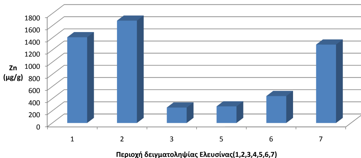
Διάγραμμα 62 - Παράρτημα 2.1 Δειγματοληψία Μαΐου 2010 στον Κόλπο της Ελευσίνας Συγκεντρώσεις ψευδάργυρου
